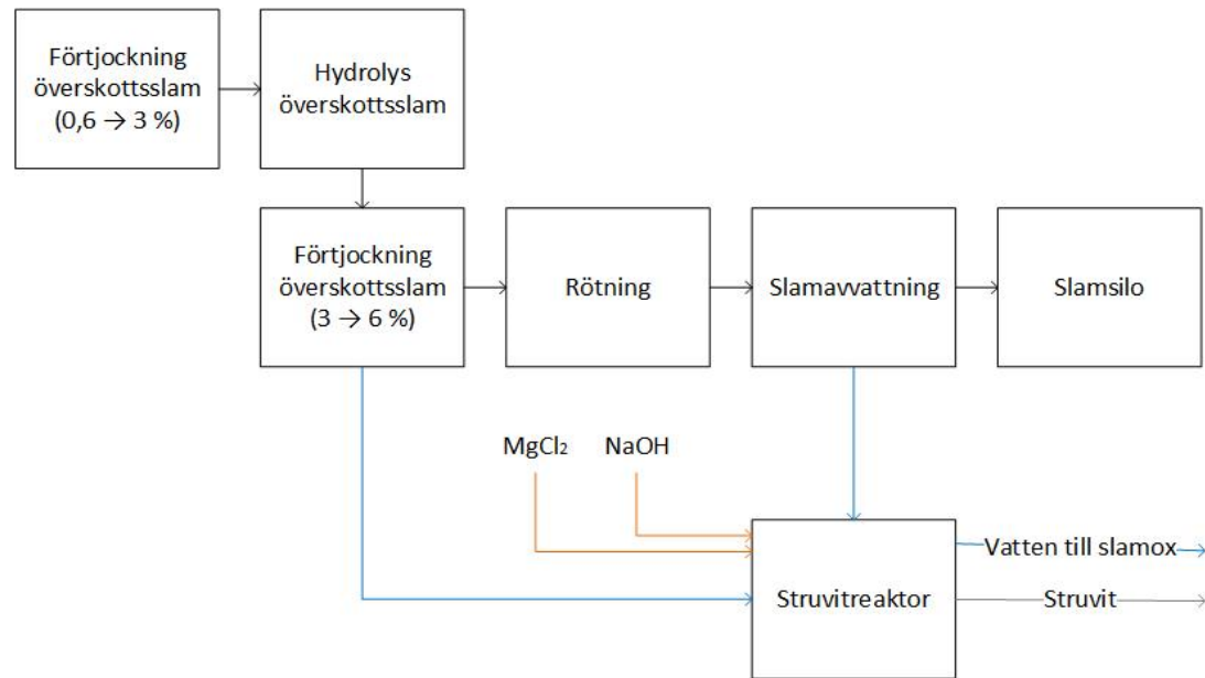
Figur 3.4 Flödesschema över fosforåtervinningsprocessen med utfällning av struvit från rejecktatten.
