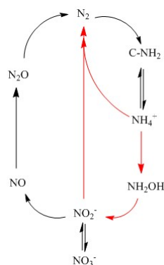
Figur 2.3: De röda pilarna representerar kväverening genom deammonifikation. Ny process som kanske skall införas på Ryaverket. Kvävefixering sker inte på avloppsreningsverk.
